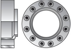
Kolnierz kompaktowy
