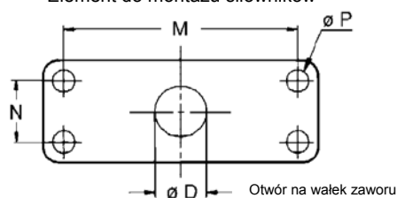
Element do montażu siłowników
