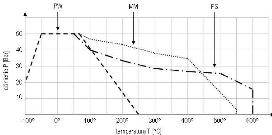
Diagram P - T dla uszczelnień PW / MM / FS DN 50 – DN 100
