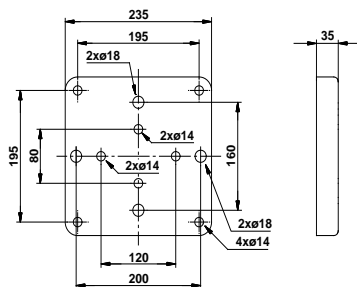
Rys. 29 Płyta montażowa do pompy UPE
