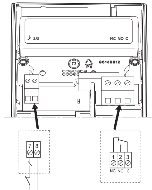
Rys. 34 Podłączenie modułu przekaźnikowego
