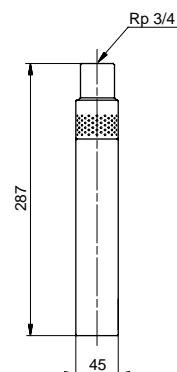
Fig. 6 MP 1 dimensions
