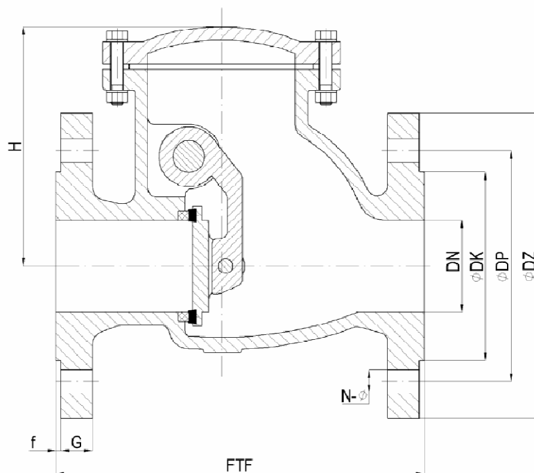
Rys. Klapa zwrotna z rewizją typ KZR.
