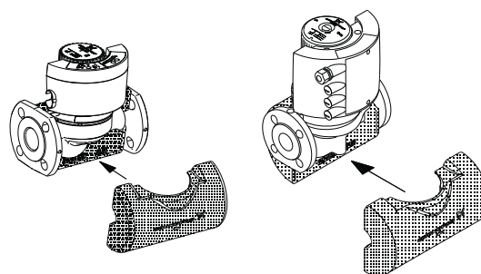
Rys. 29 Montaż okładzin na pompie MAGNA
