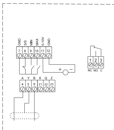
Rys. 31 Podłączenie modułu GENI
