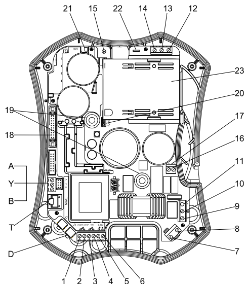
Rys. 24 Zaciski wewnątrz skrzynki zaciskowej pompy UPE(D).
