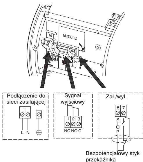
Rys. 23 MAGNA 32-120, 40-120, 50-120, 65-120, 50-60, 65-60. Podłączenie elektryczne do sieci zasilającej.
