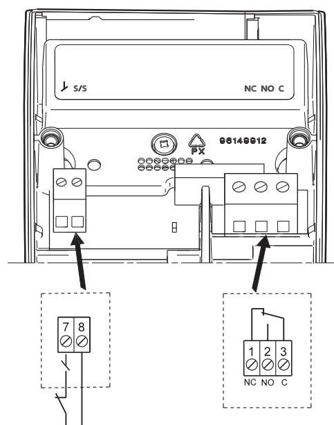
Rys. 32 Podłączenie modułu przekaźnikowego
