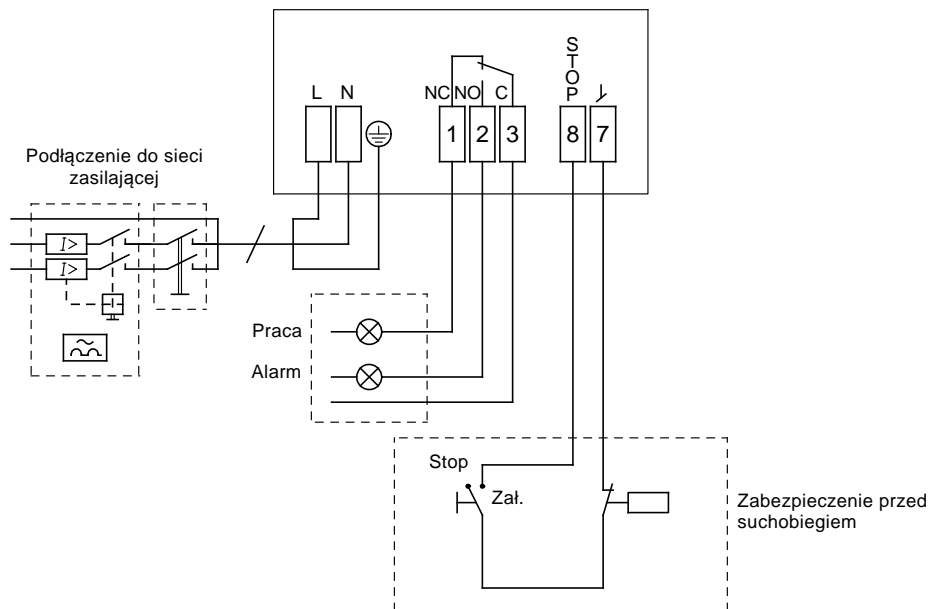
Rys. 25 Przykład połączeń dla pompy MAGNA
