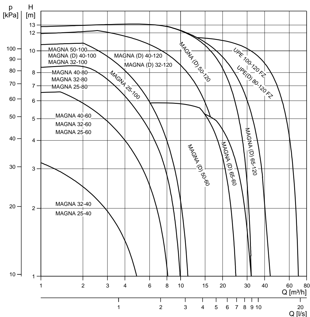
Rys. 2 Pola pracy
