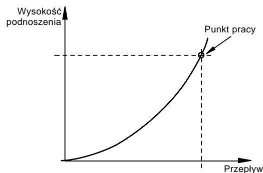
Rys. 3 Charakterystyka instalacji
