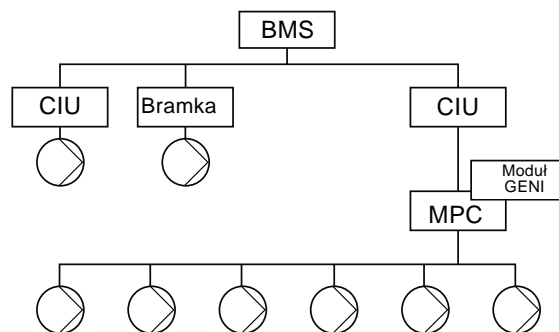
Rys. 15 UPE Seria 2000 FZ w systemie BMS
