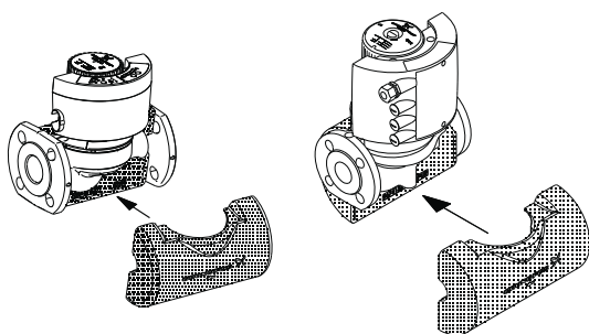
Rys. 28 Montaż okładzin na pompie MAGNA
