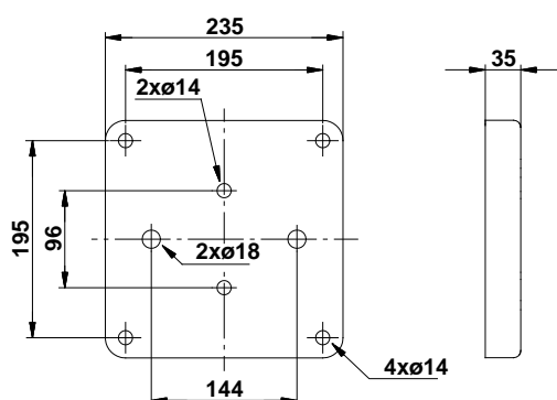
Rys. 27 Płyta montażowa do pompy MAGNA
