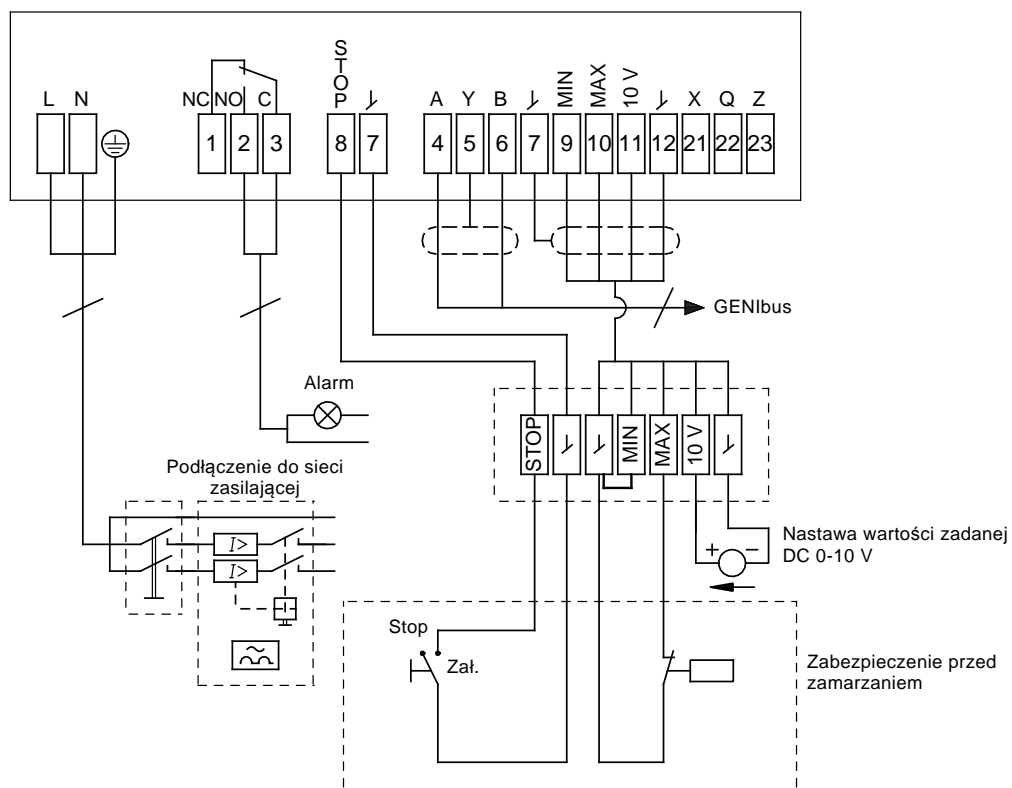
Rys. 26 Przykład połączeń dla pompy MAGNA z modułem GENI
