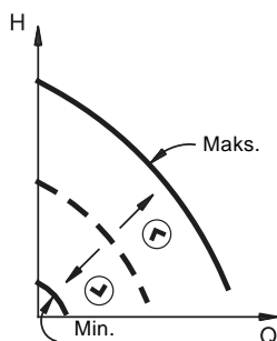
Rys. 8 Charakterystyka stała
