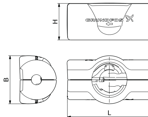
Rys. 30 Rysunek wymiarowy okładzin termoizolacyjnych do klimatyzacji
