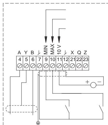
Rys. 33 Podłączenie modułu GENI
