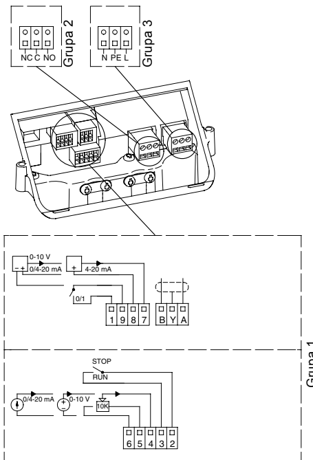
Rys. 31 Pompy TPE, schemat połączeń, silnik 1-fazowy
