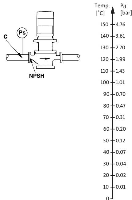
Rys. 36 Minimalne ciśnienie wlotowe
