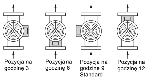
Rys. 27 Możliwe pozycje skrzynki zaciskowej
