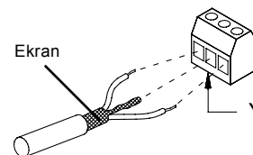
Rys. 30 Podłączenie komunikacji bus do TPE, TPED
